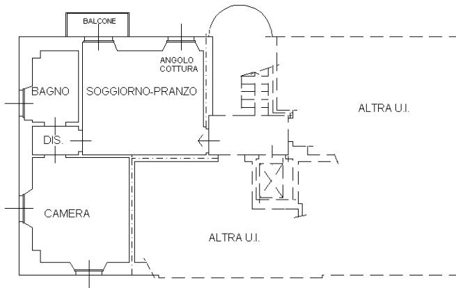
PIANO PRIMO H=ml.3.20
