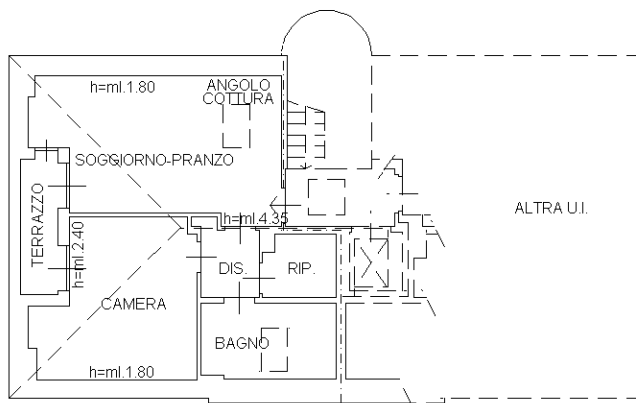
PIANO SECONDO H.MEDIA= ml.3.07
